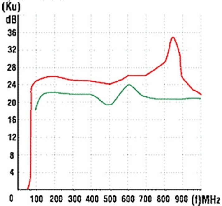
Wykres wzmacnienia:
