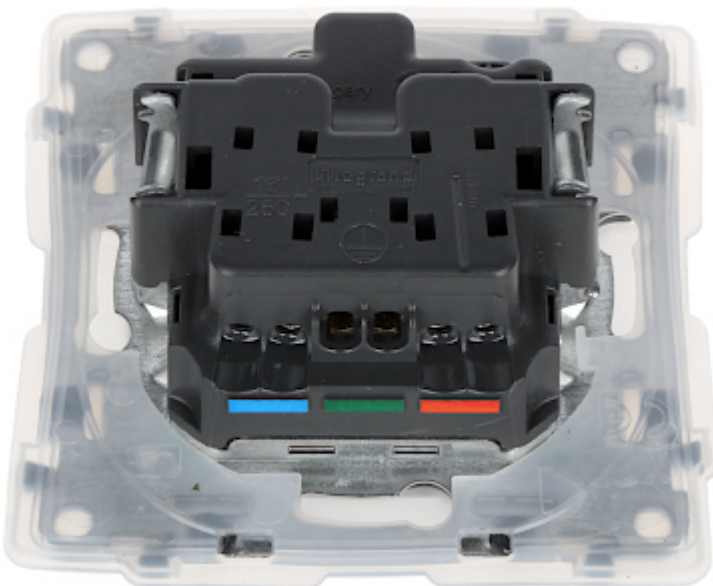
Widok złącz:
