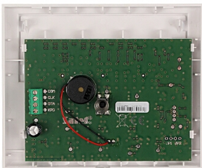
Widok od strony mocowania:
