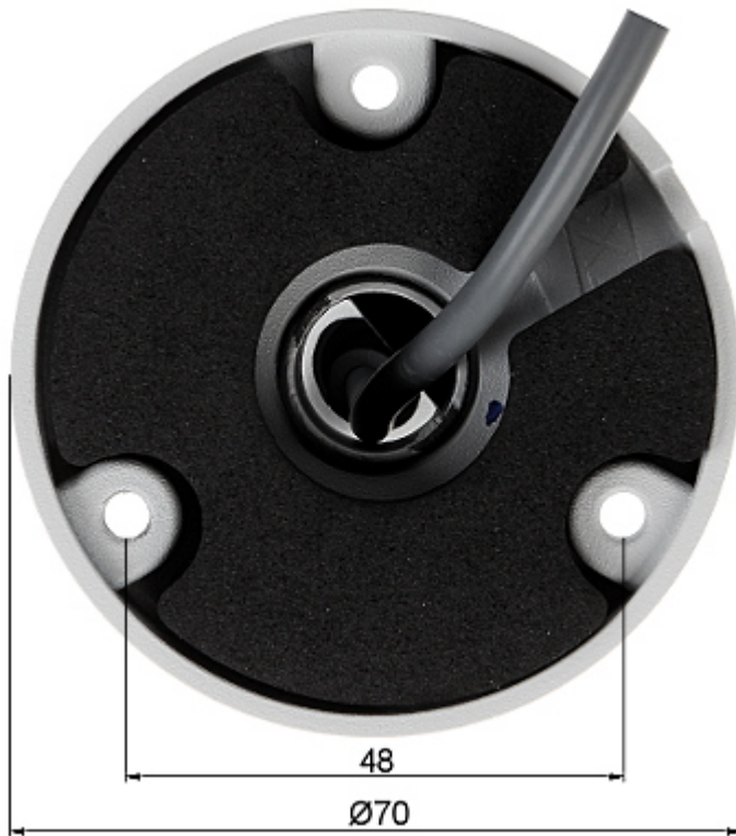
Wymiary kamery:
