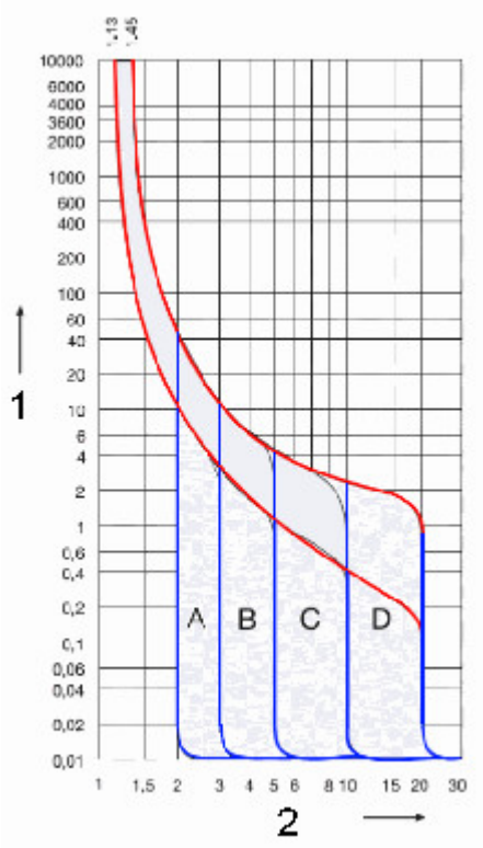
Charakterystyka wyzwalania:
