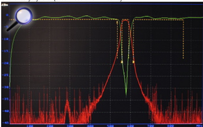
Charakterystyka częstotliwościowa zwrotnicy:
