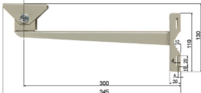
Wymiary uchwytu:
